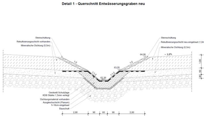
Bild 1: Planungsskizze
