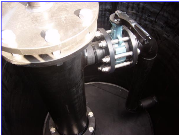
Bild 2: Deponiegasbrunnen Detail
